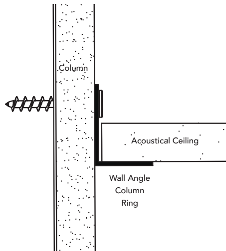
ACOUSTICAL/DRYWALL CROSS SECTION)
